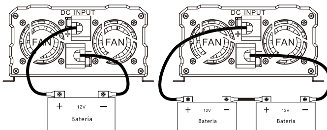
Diagrama del inversor de 12V conectado a la batería
